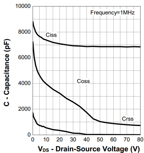
11. Capacitance
